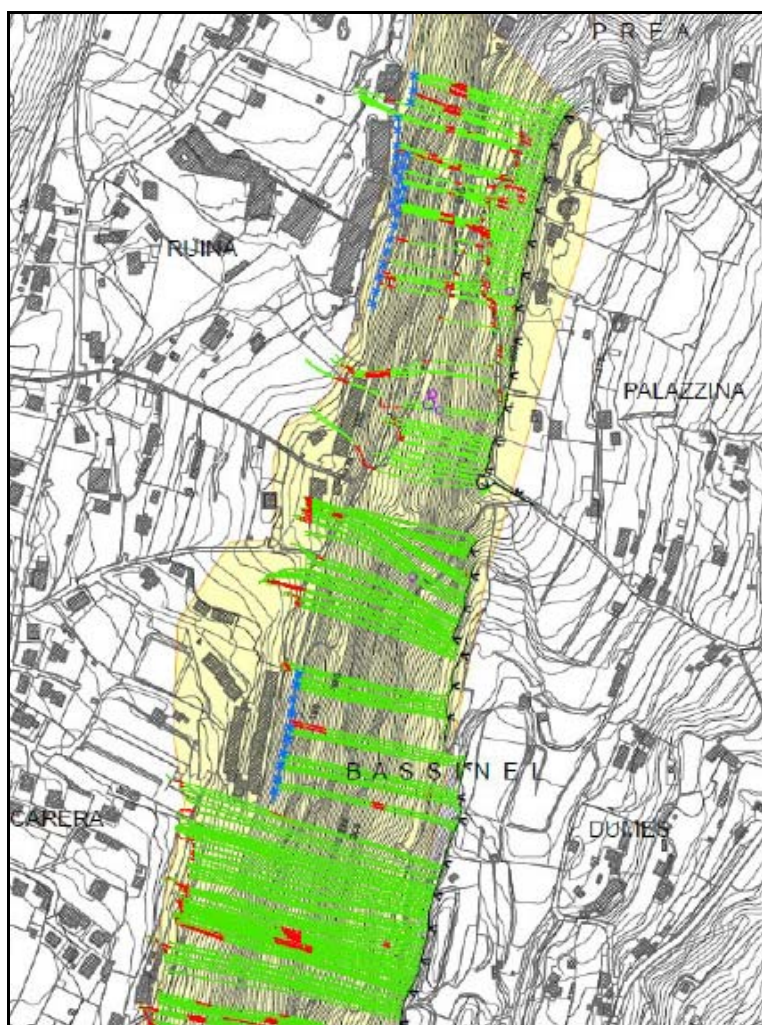
Fig. 8 – Calcolo degli scendimenti dei blocchi in presenza di opere di protezione tra le loc. Ruina e Carera.
