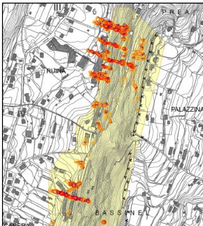
Fig. 7 – Calcolo delle altezze massime delle traiettorie dei massi tra le loc. Ruina e Carera.
