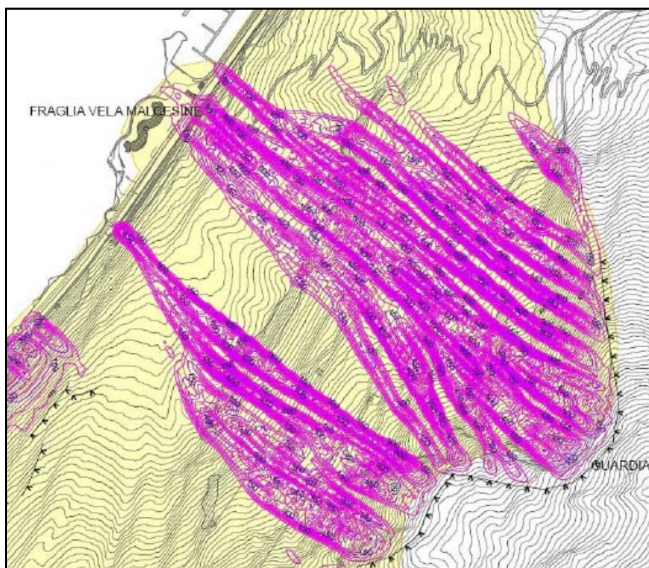
Fig. 6 – Calcolo delle energie specifiche massime nella zona delle Fraglie (area SAR_2).
