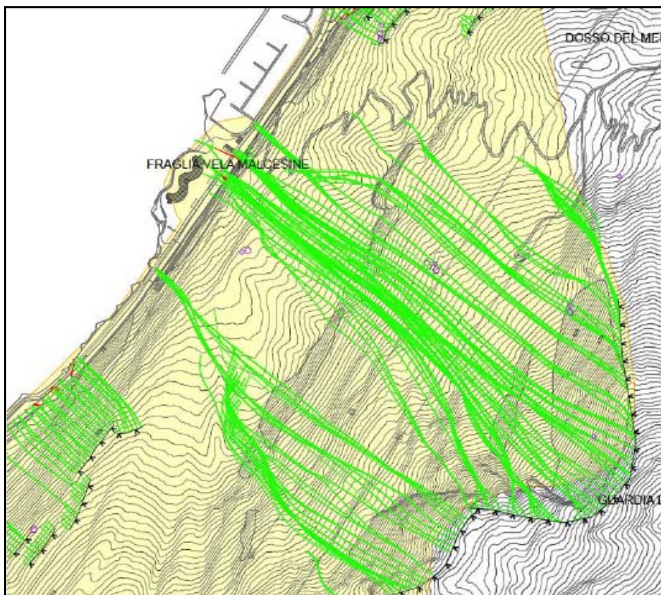
Fig. 5 – Calcolo dei scendimenti dei blocchi in assenza di opere di protezione.
